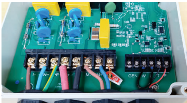
Instalação do controlador sem o uso do sensor de poço.
