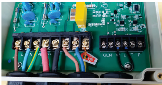
Instalação do controlador sem uso de sensores de nível.
